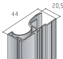
Profil S12
