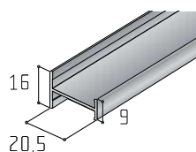
Profil H 9/16
