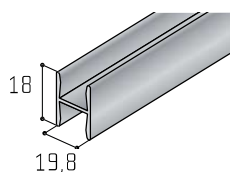
Profil H kov
