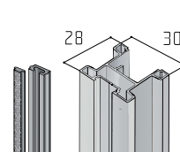
Profil S19*
