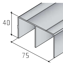
Profil S05
