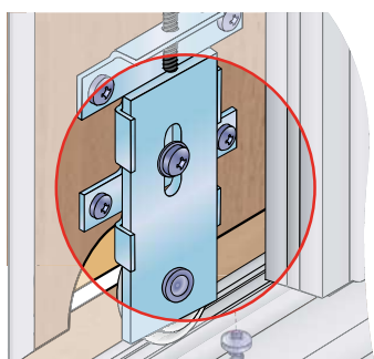
Dolní vozík
