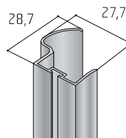
Profil S13B
