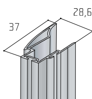
Profil S04N
