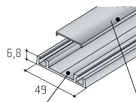
Profil S06 N krycí Profil S06 N
