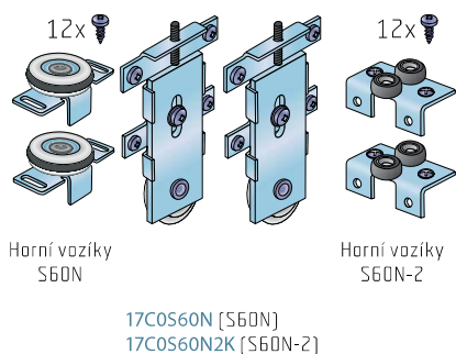
Sada S60N / Sada S60N-2
