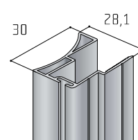
Profil S14
