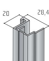
Profil S08
