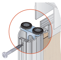
Montáž horního vozíku
