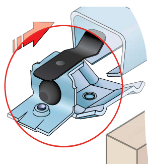
Montáž brzdy
